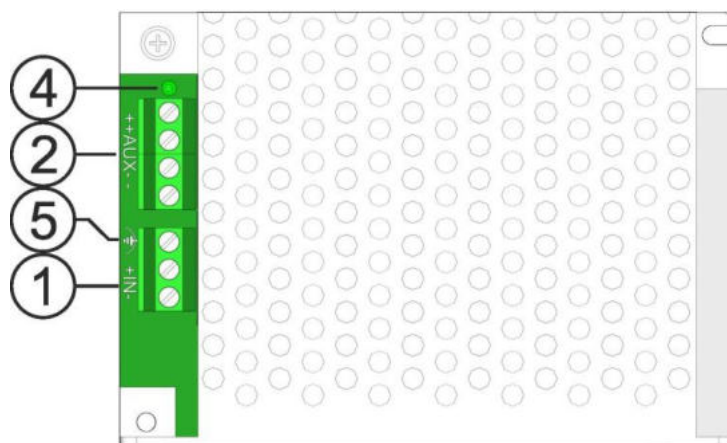
Obr. 2c. Pohled na konvertorový modul DCDC-12V5A-SE; DCDC-12V4A-SE; DCDC-24V2A-SE.
