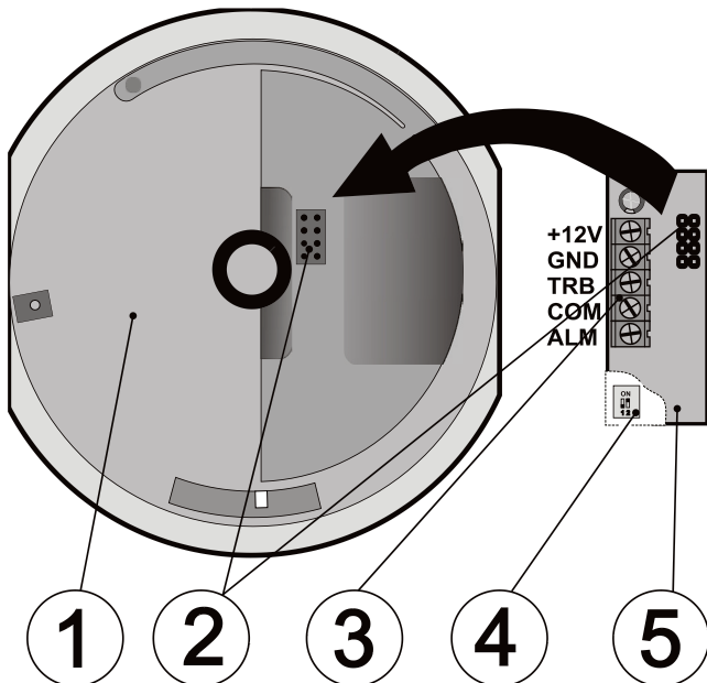
Obrázek: 1 – Detektor Ei208(D)W, 2 – systémový konektor pro připojení s Ei208(D)W, 3 – svorkovnice, 4 – přepínače DIP pro volbu funkce výstupů (na spodní straně modulu), 5 – drátový modul GS-208-CO
