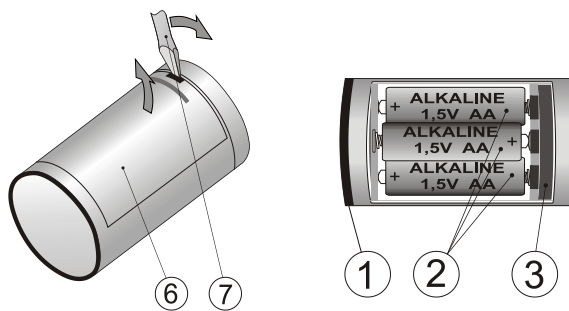
Obrázek 3: 1 – Signálka; 2 – Baterie; 3 – Pojistný kroužek 6 – Kryt baterií; 7 – Pomocný nástroj (šroubovák)
