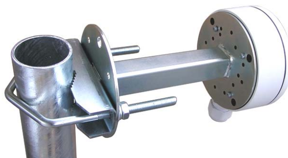
HIK170N + Z5V105 + DS-1280ZJ-DM18
