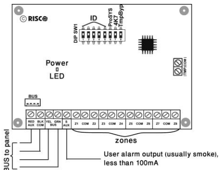
Obrázek 3-2: Deska expandéru zón a zapojení
