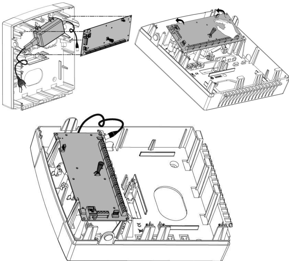
Obrázek 2-4 Umístění hlavní jednotky
