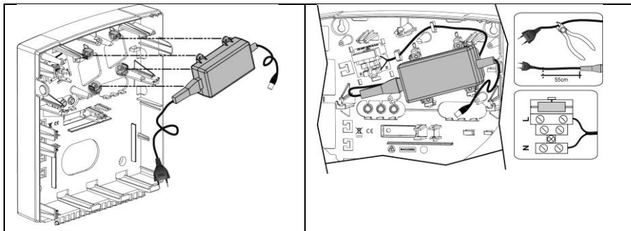
Obrázek 2-3 Umístění AC adaptéru a pojistky
