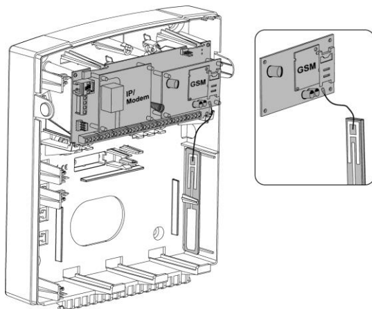
Obrázek 2-10 Umístění GSM/GPRS modulu a antény
