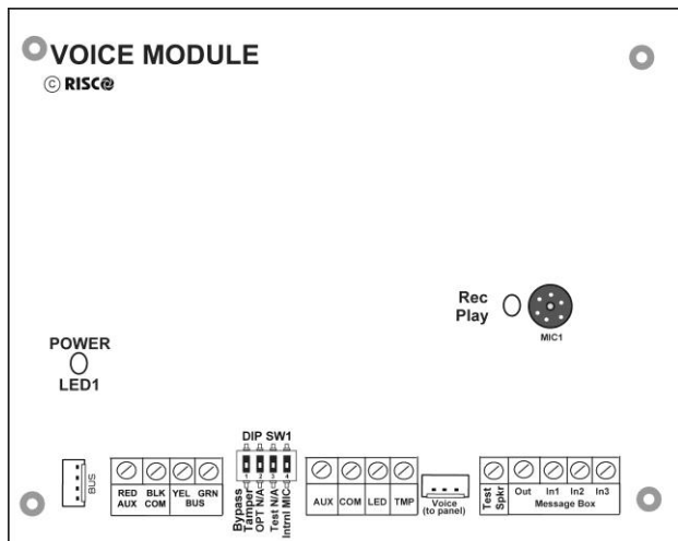
Obrázek 3-11: Deska hlasového modulu
