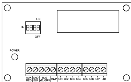
Obrázek 3-5: Modul výstupů EO8
