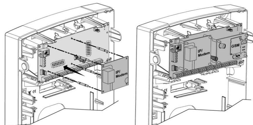
Obrázek 2-11 Umístění IP modulu
