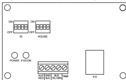
Obrázek 3-6: Modul výstupů X-10
