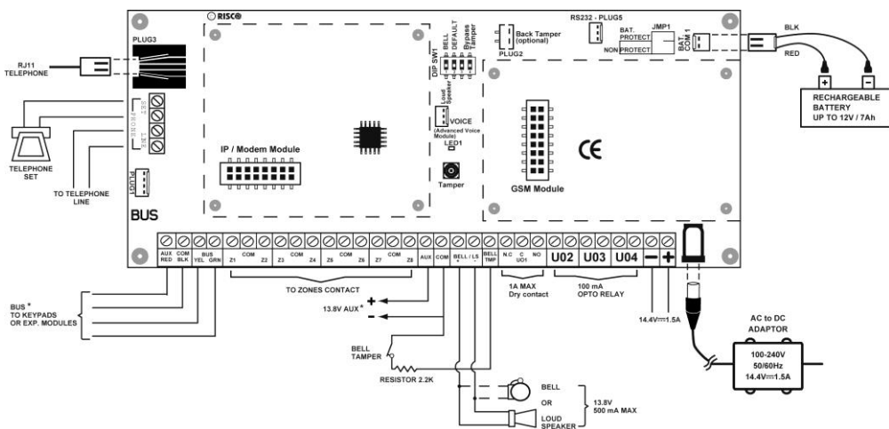
Obrázek 2-5: Zapojení hlavní jednotky
