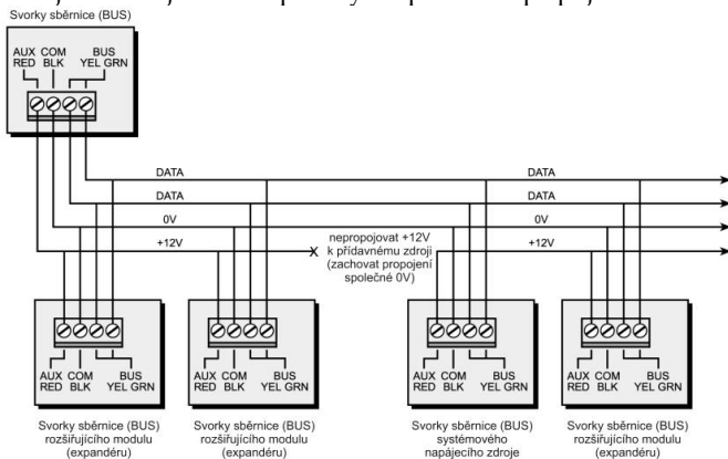
Obrázek 3-1: Svorky připojení sběrnice
