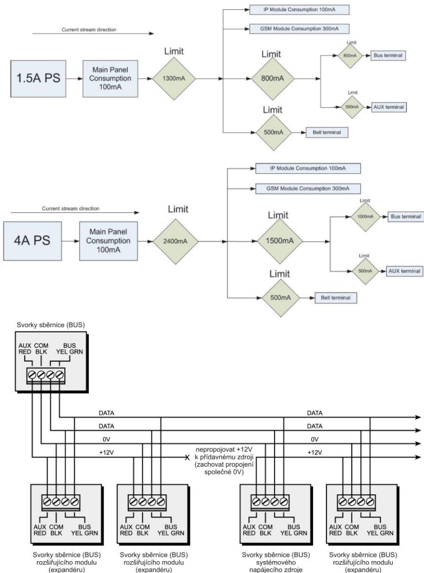
Obrázek 2-7: Svorky připojení sběrnice
