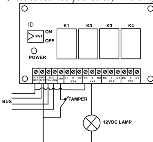
Obrázek 3-4: Modul výstupů UO4 (s příkladem zapojení UO4)
