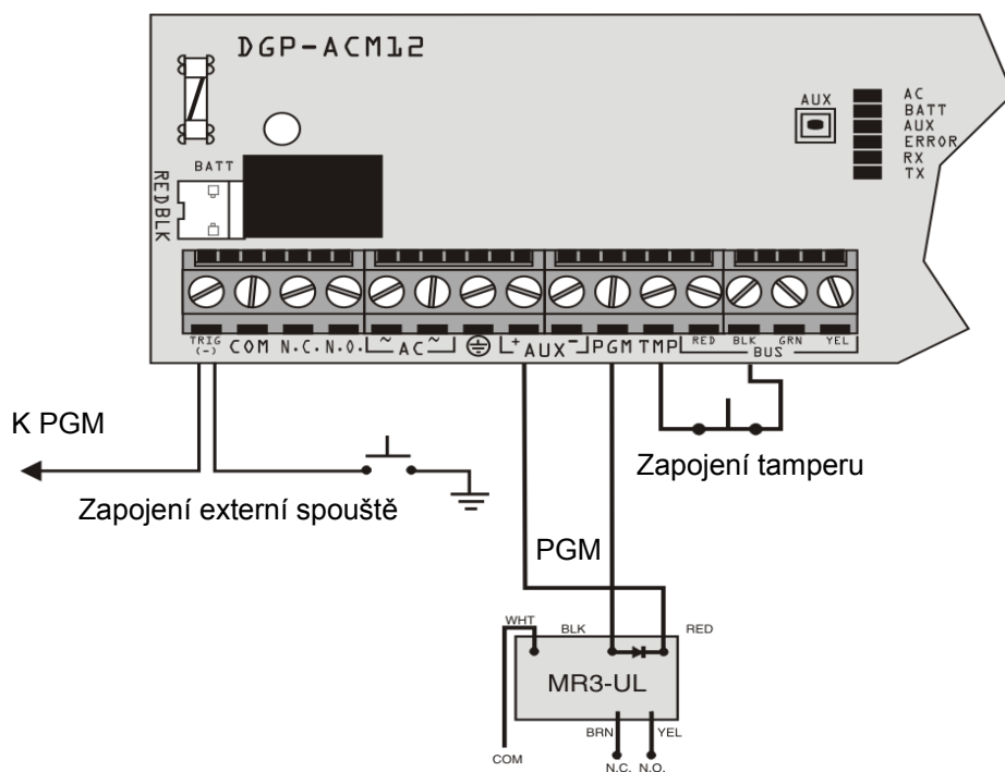
Obr. 2: Další zapojení
