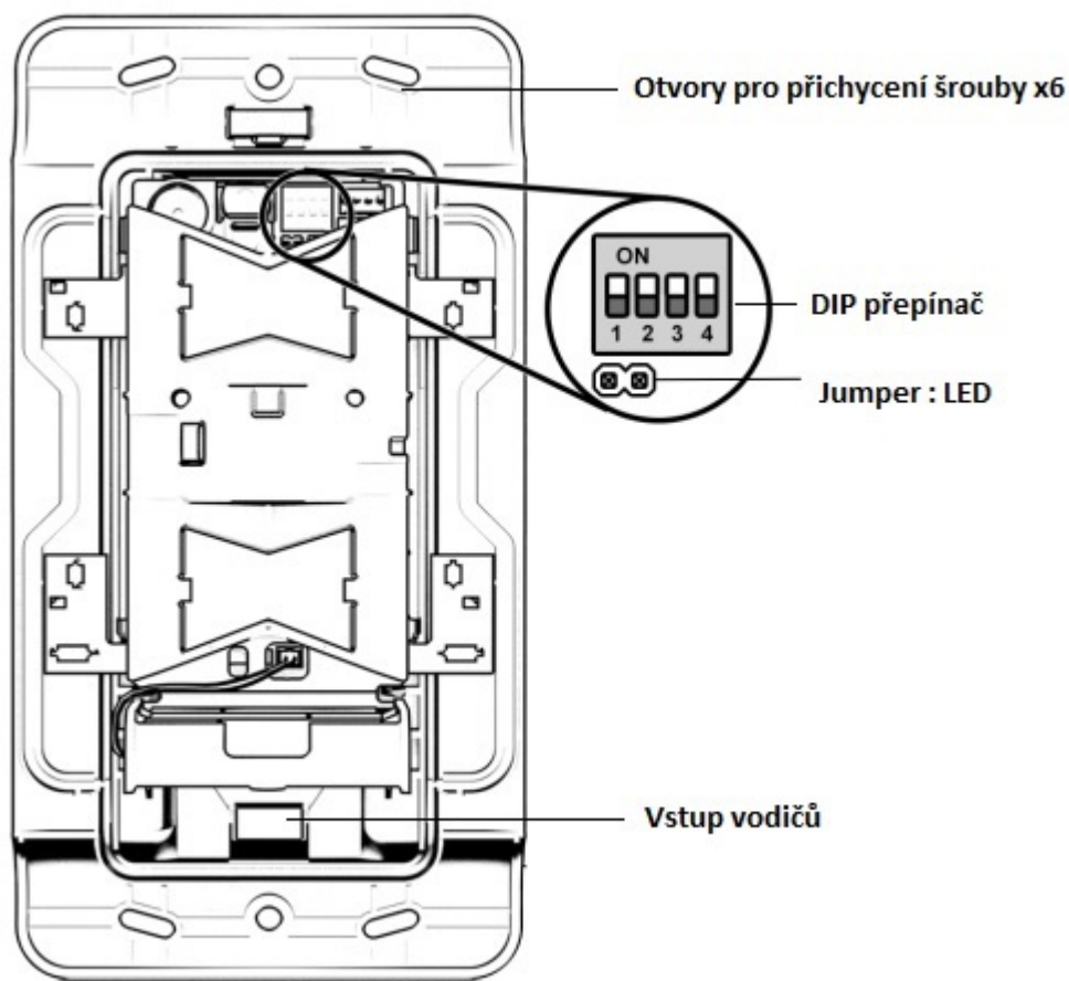
Obrázek 1 – Vnitřek detektoru
