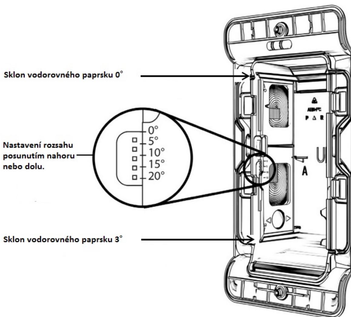
Obrázek 2 - nastavení sklonu a dosahu detektoru
