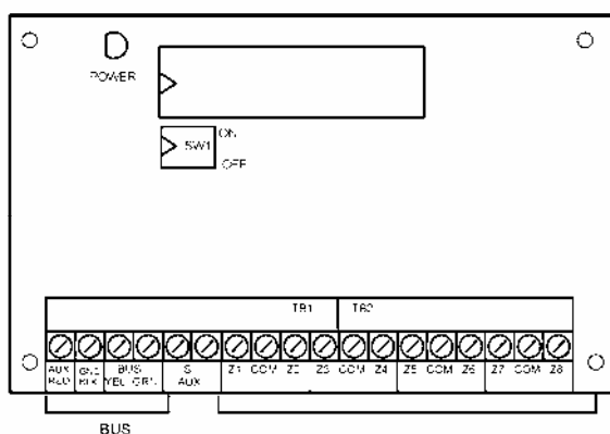
Obr. 3-3: Rozšiřující modul zóny ZE8 (na obrázku je příklad typického připojení)
