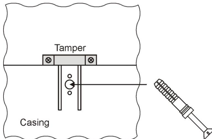
Obr. 4. Montáž držáku tamperu proti sabotáži.
