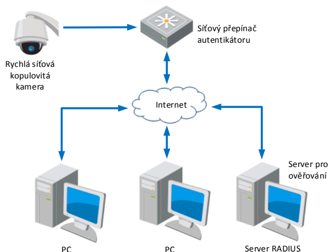
Obrázek 6–17 Chráněná síť LAN
